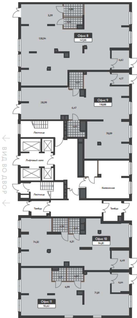
1 этаж
