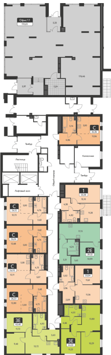
Первый этаж
